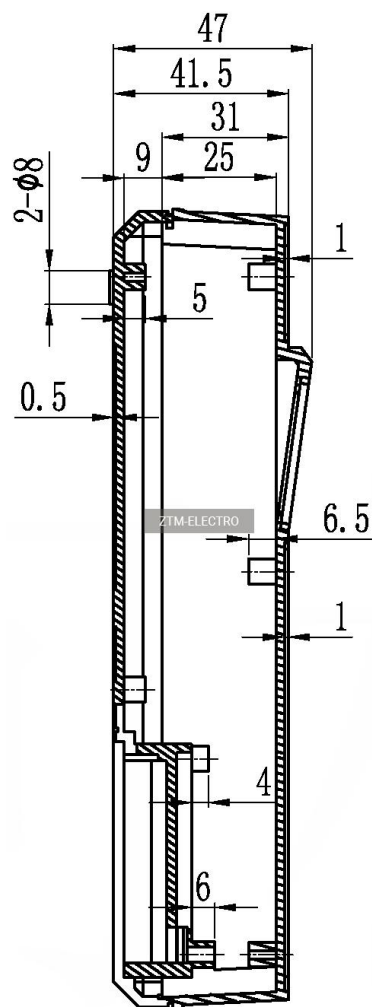
Section A-A
